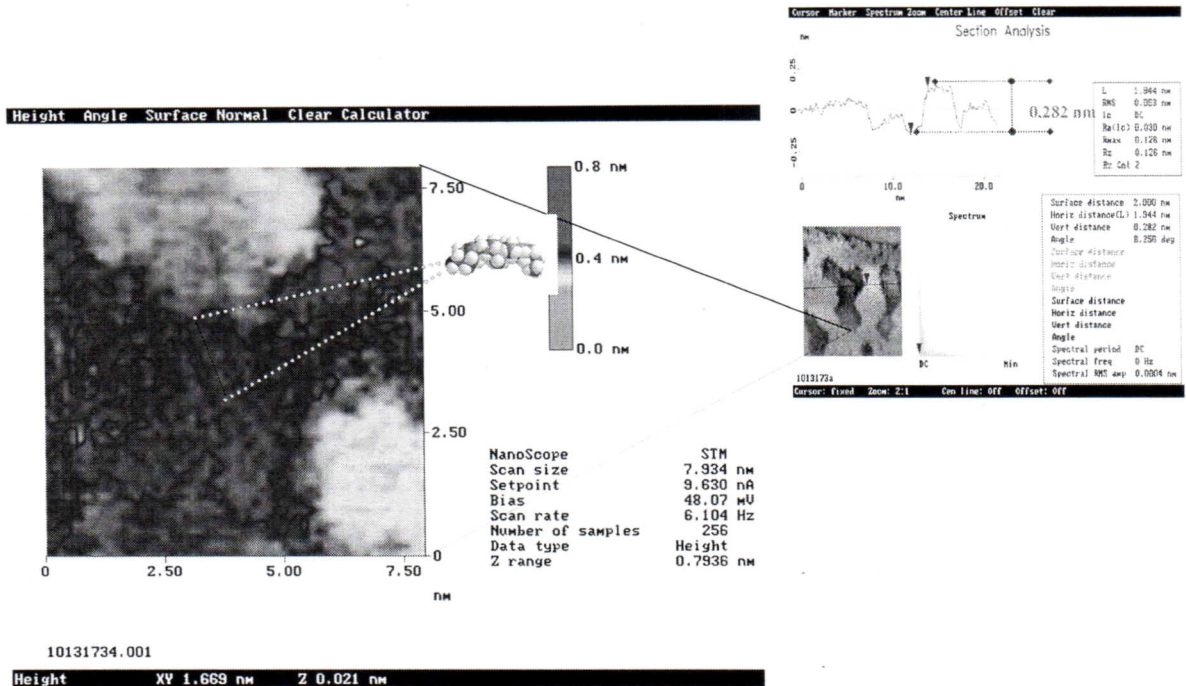
Figura 4. STM imagen de alta resolución de capas de moléculas de colesterol monohidratado ( 2 \times 10^{-4} M) en agua y adsorbidas a temperatura ambiente sobre Au (111). Esta imagen muestra capas de colesterol, con posibilidad de identificar moléculas individuales de colesterol.
